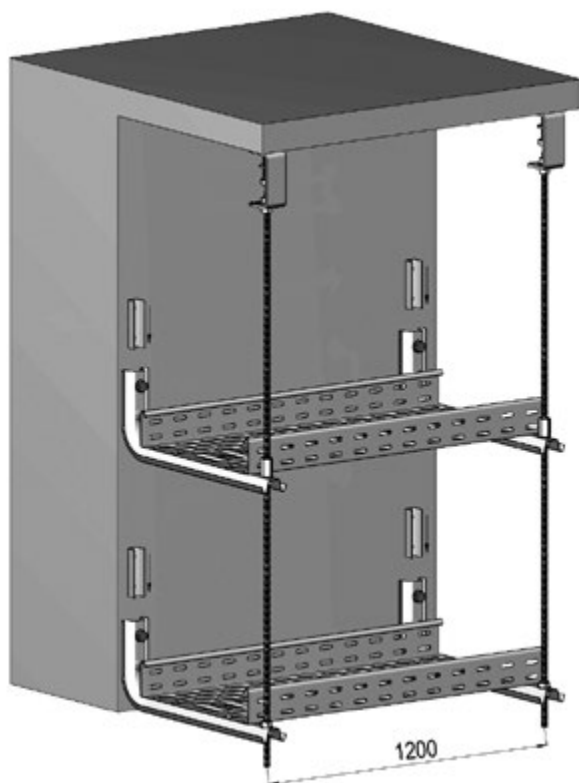
Oldalfali rögzítés, kiegészítő menetes szásas biztosítással mennyezetre
